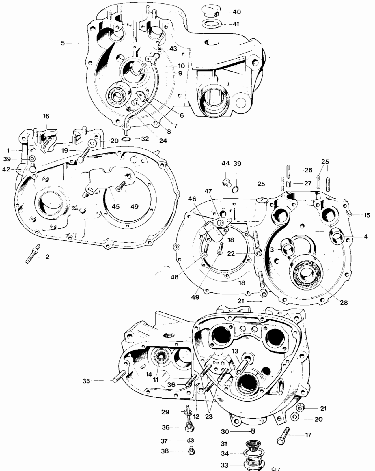
Fig. 2. CRANKCASE
