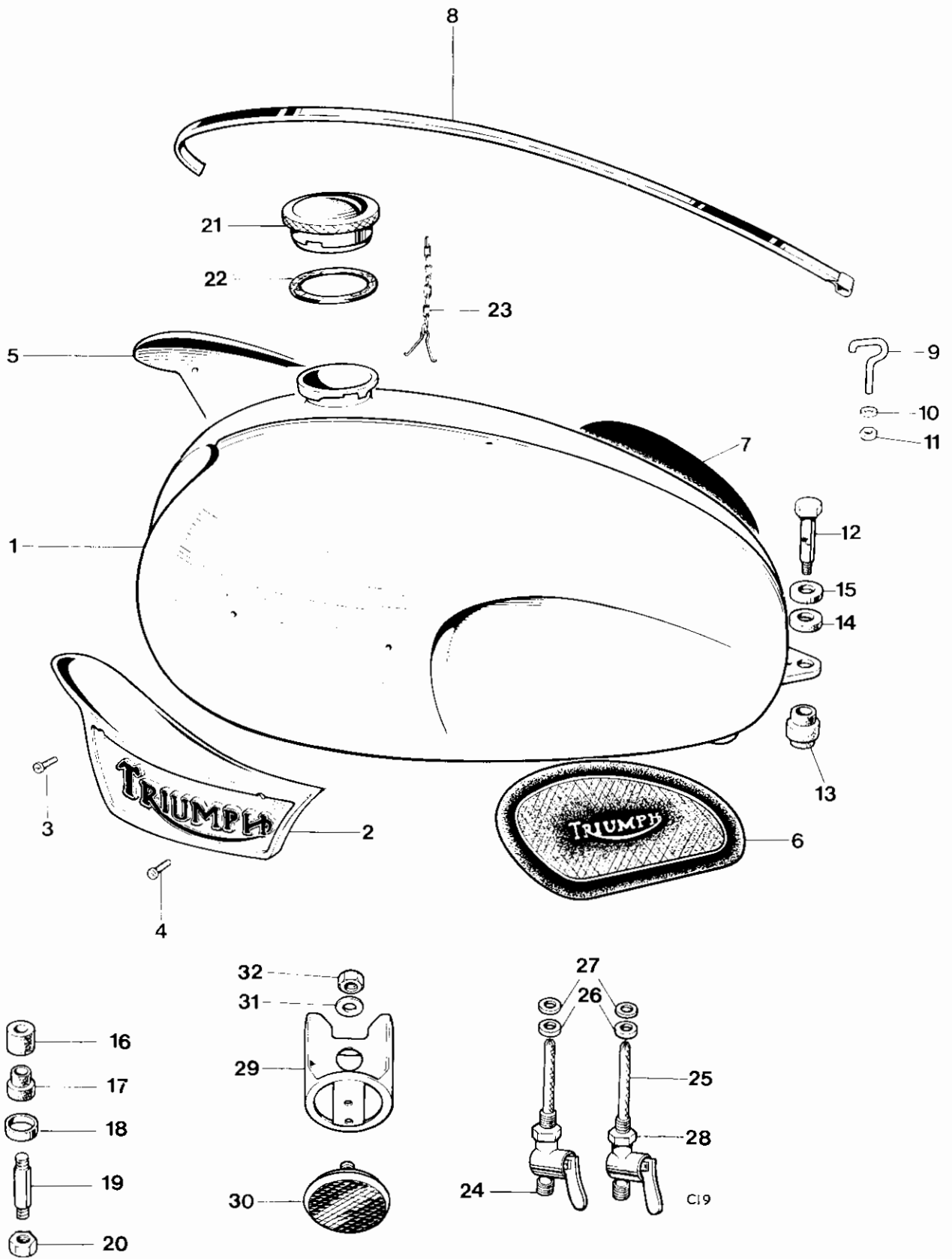
Fig. 27. GAS TANK
