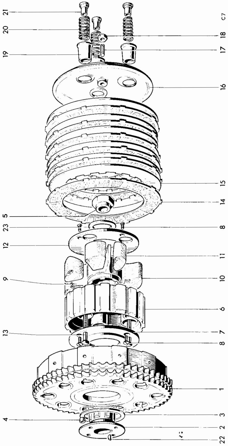
Fig. 13. CLUTCH
