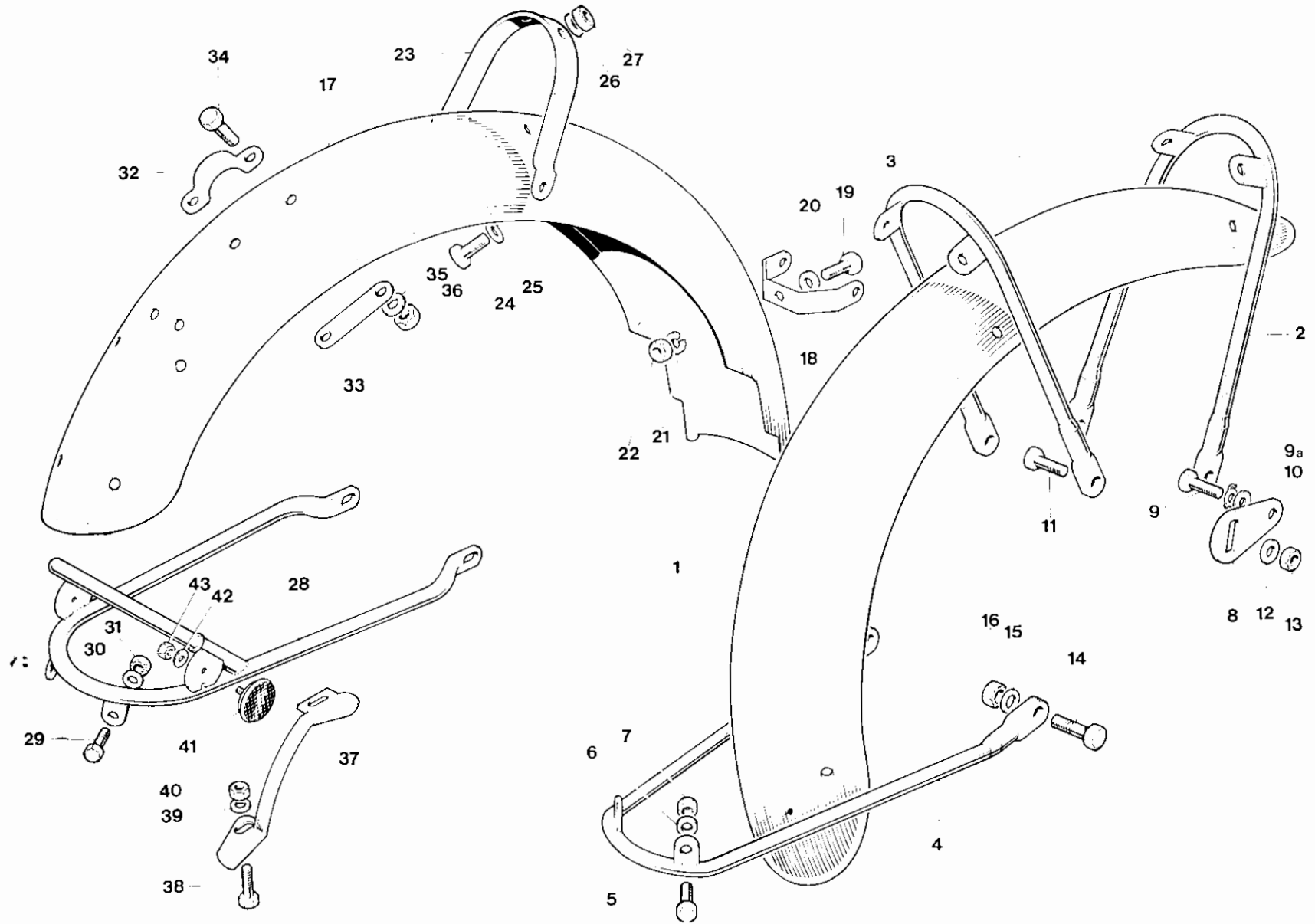
Fig. 24. FENDERS
